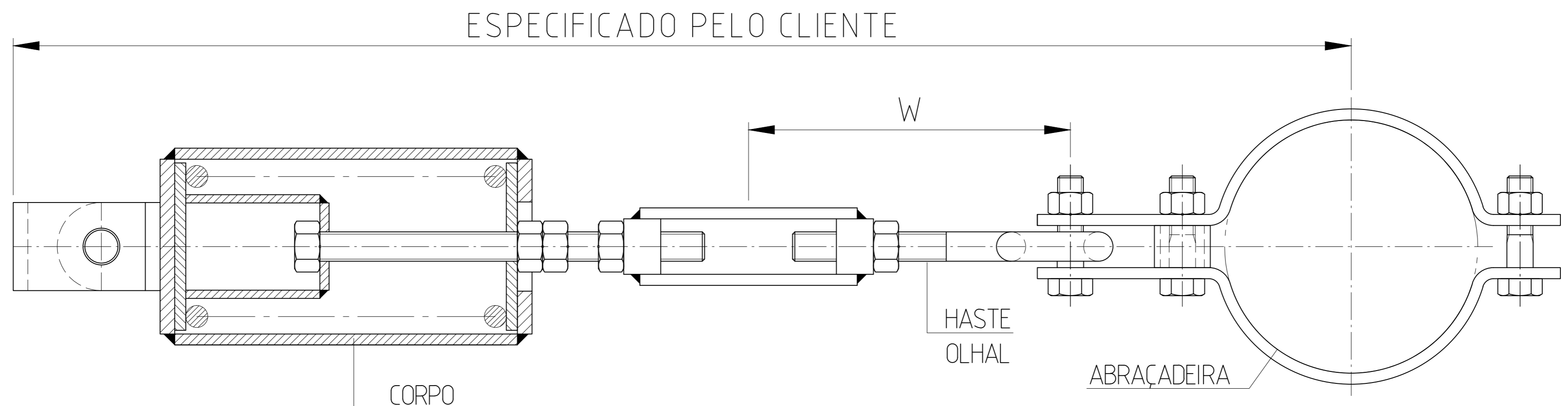
FIGURA VCBO RECOMENDADO QUANDO A DIMENSÃO W É IGUAL A 610mm OU MENOR
