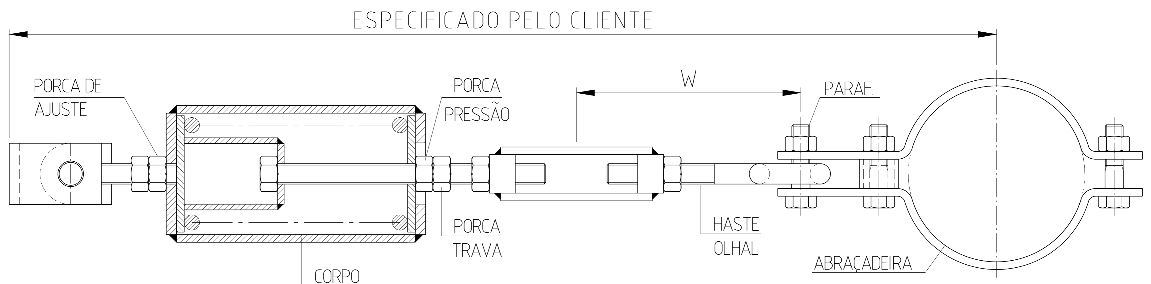
FIGURA VCAO RECOMENDADO QUANDO A DIMENSÃO W É IGUAL A 610mm OU MENOR
